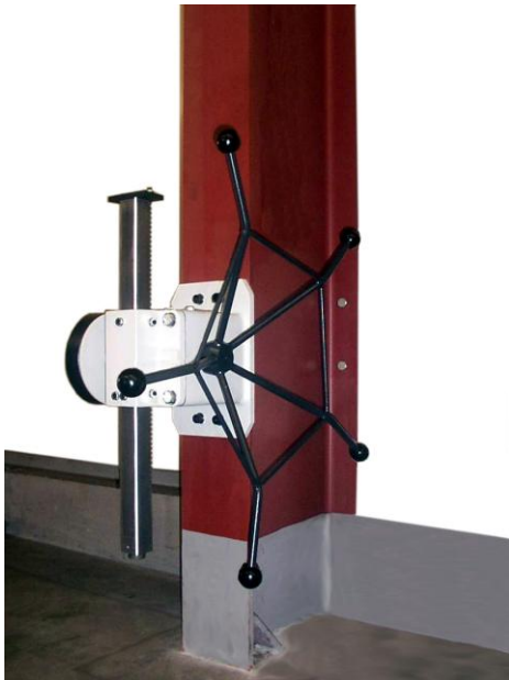
Räumpresse T5 für Wand – bzw. Kranbefestigung
